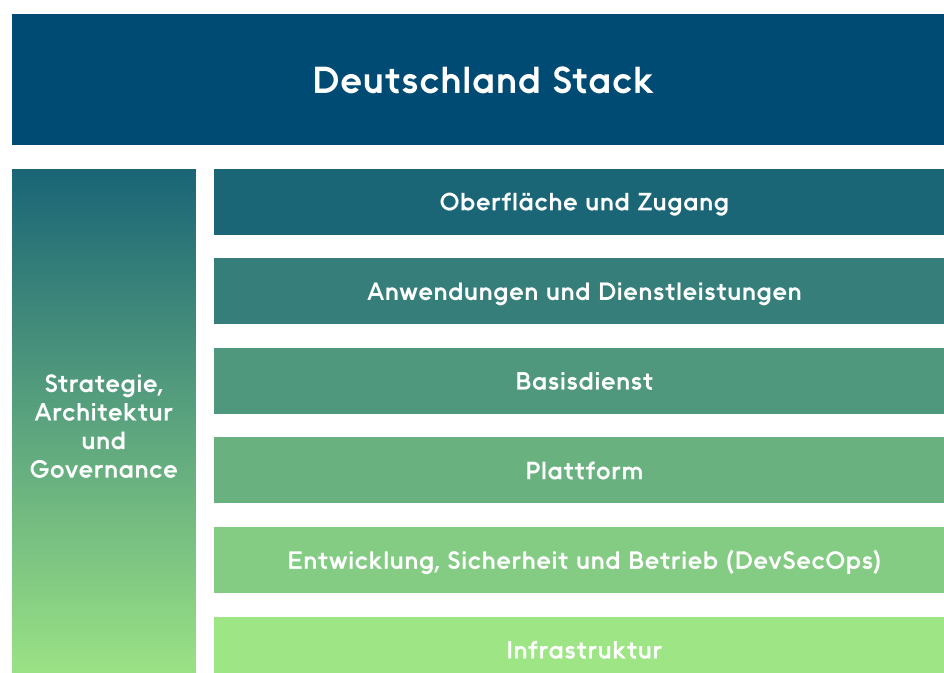
Abb. 04-4: Deutschland Stack
