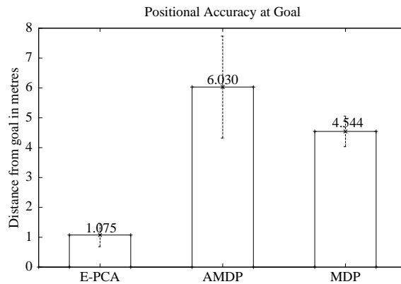
(d) Policy Performance
